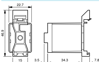
Top 35 mm rail (EN 50022) adaptor for 55.32, 55.33, 55.34
