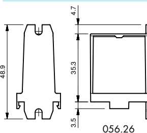
Top 35 mm rail (EN 50022) adaptor for 55.32, 55.33, 55.34
